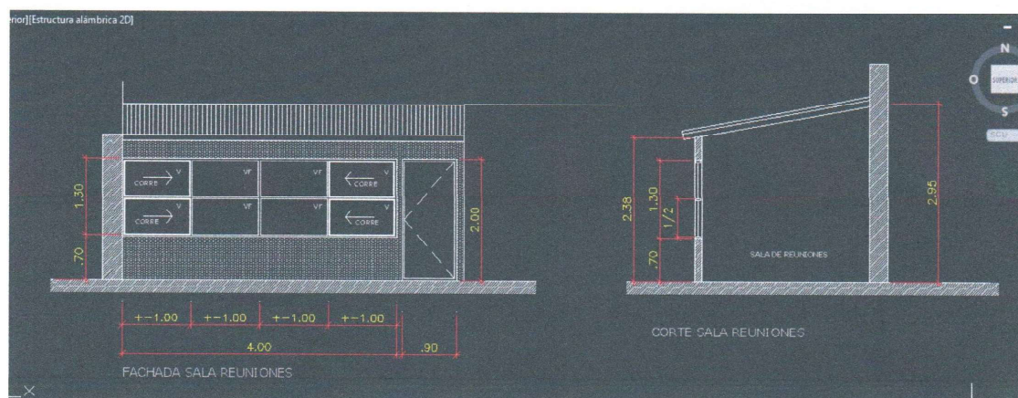
FACHADA SALA REUNIONES NUEVAS DEPENDENCIAS DESAM
